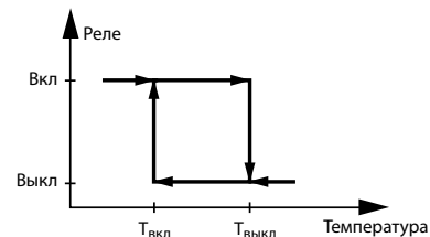
Рис. 10. Гистерезис работы.
